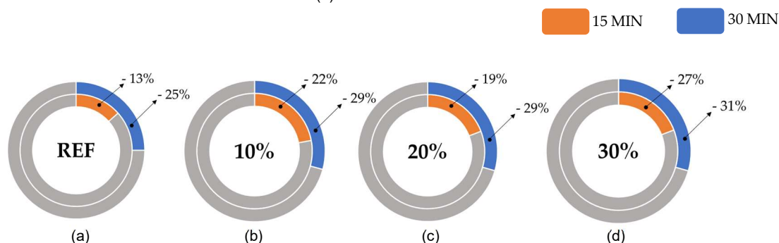
Figura 1: Comparativo de redução de consistência com o passar do tempo: (a) Argamassa referência, (b) 10% RCC, (c) 20% RCC e (d) 30% RCC
