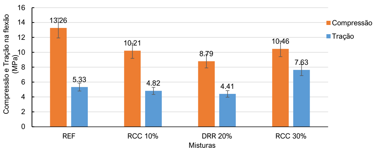
Figura 2: Comparativo de Variação de Resistência Média à Tração na Flexão e Compressão
