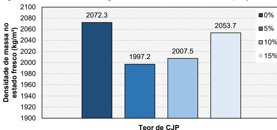
Figura 4: Densidade de massa das argamassas no estado fresco, sem e com incorporação de CJP.
