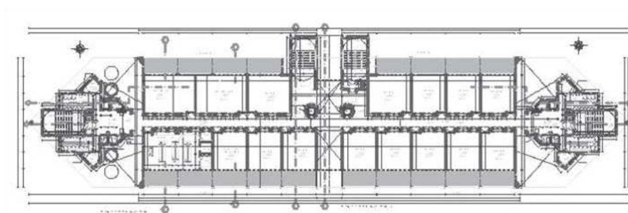
Figura 1 – Planta do pavimento tipo da edificação em análise.
