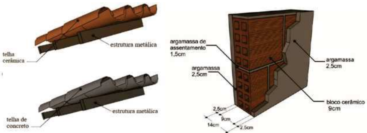
Figura 1 – Detalhes esquemáticos da cobertura e paredes dos protótipos (Fonte: Imagem baseada no modelo do livro SELO CASA AZUL, 2010).
