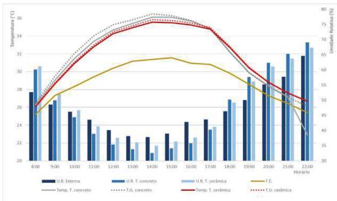
Figura 5 – Dados relativos às umidades relativa médias internas e externa, temperaturas médias internas e externas e temperaturas de globo (Autores, 2021).
