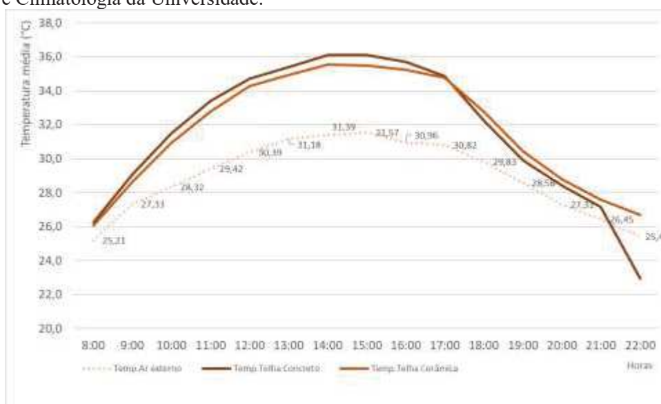
Figura 4 – Dados relativos às temperaturas médias internas dos protótipos (com telha cerâmica e telha concreto) e temperatura externa dos dias 23, 24 e 25 de junho de 2020 (Autores, 2021).
