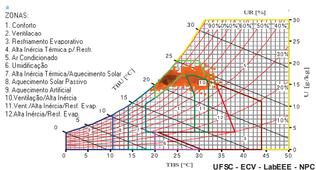
Figura 24 – Carta bioclimática de verão para Maceió
