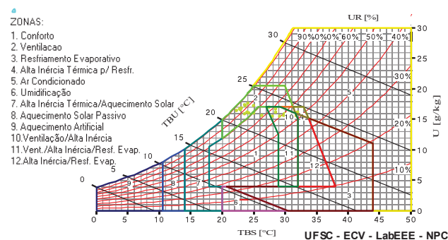
Figura 25 – Carta bioclimática dia típico de verão para Maceió
