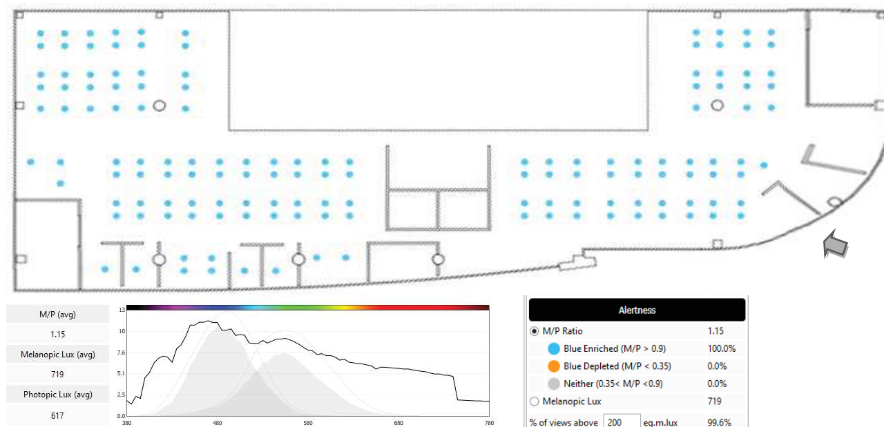
Figura 6 Resultado da simulação apenas com iluminação natural.
