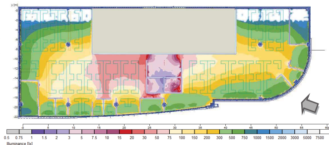
Figura 8 Simulação da iluminação natural no dia 21.03 às 9h.
