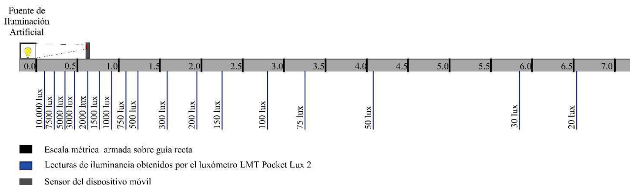
Figura 1. Esquema del arreglo experimental por medio del que se contrastaron los valores de iluminancia obtenidas por el luxómetro LMT Pocket Lux 2 y las aplicaciones instaladas en los smartphones.
