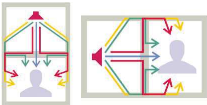
Figura 1 – Transmissão do ruído aéreo entre ambientes - retirado de ProAcústica (2013).
