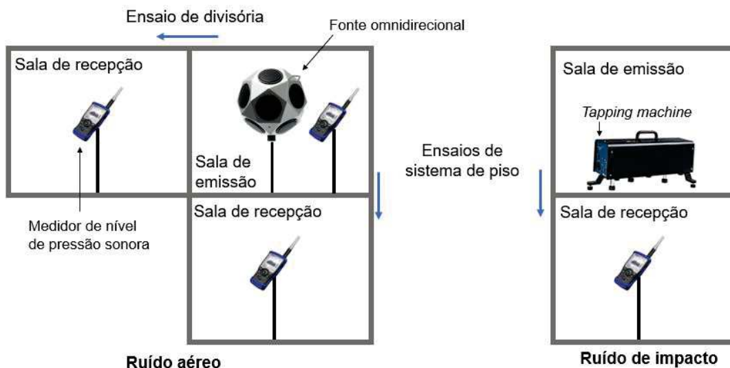
Figura 5 – Esquema simplificado dos ensaios de ruído aéreo e de impacto
