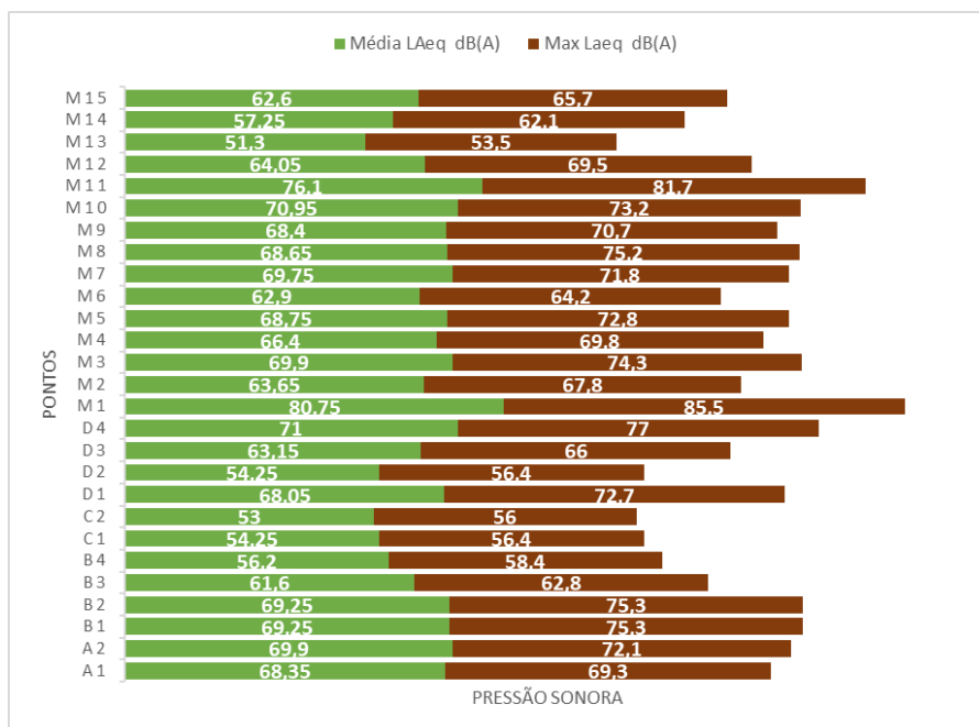
Figura 07 – Gráfico com Valores dos níveis de pressão sonora equivalentes -1 min – ponderados na Rua Maj. Carlos Del Prete (LAeq, 1min) para os levantamentos de campo no inverno.
