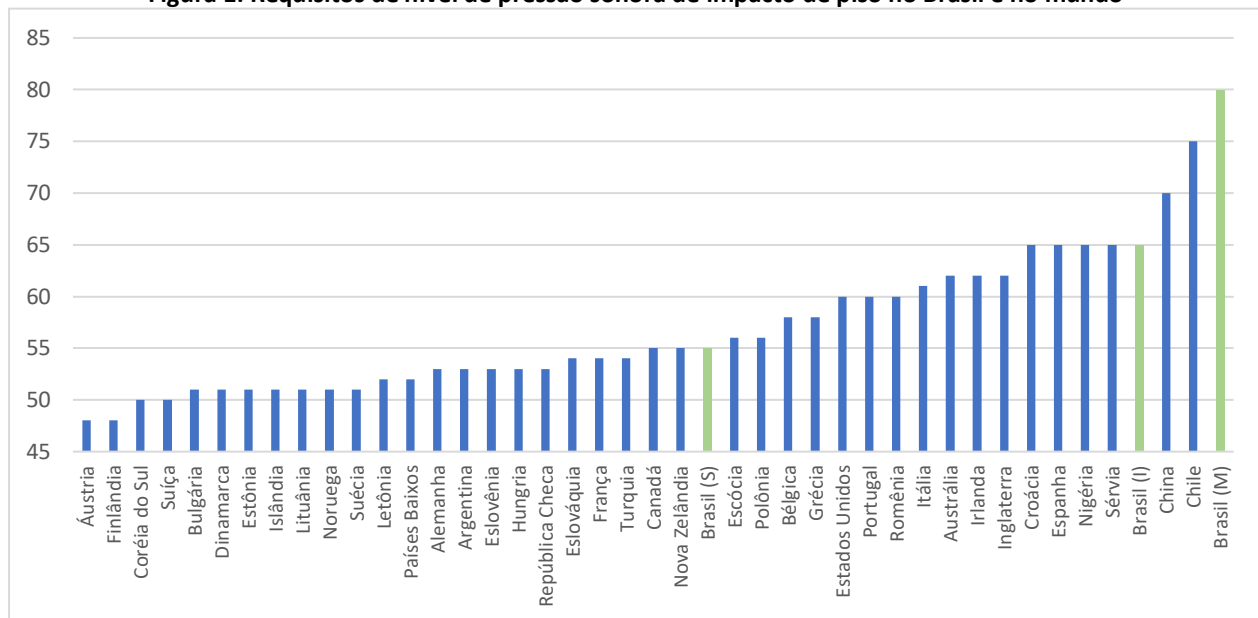
Figura 1: Requisitos de nível de pressão sonora de impacto de piso no Brasil e no mundo
