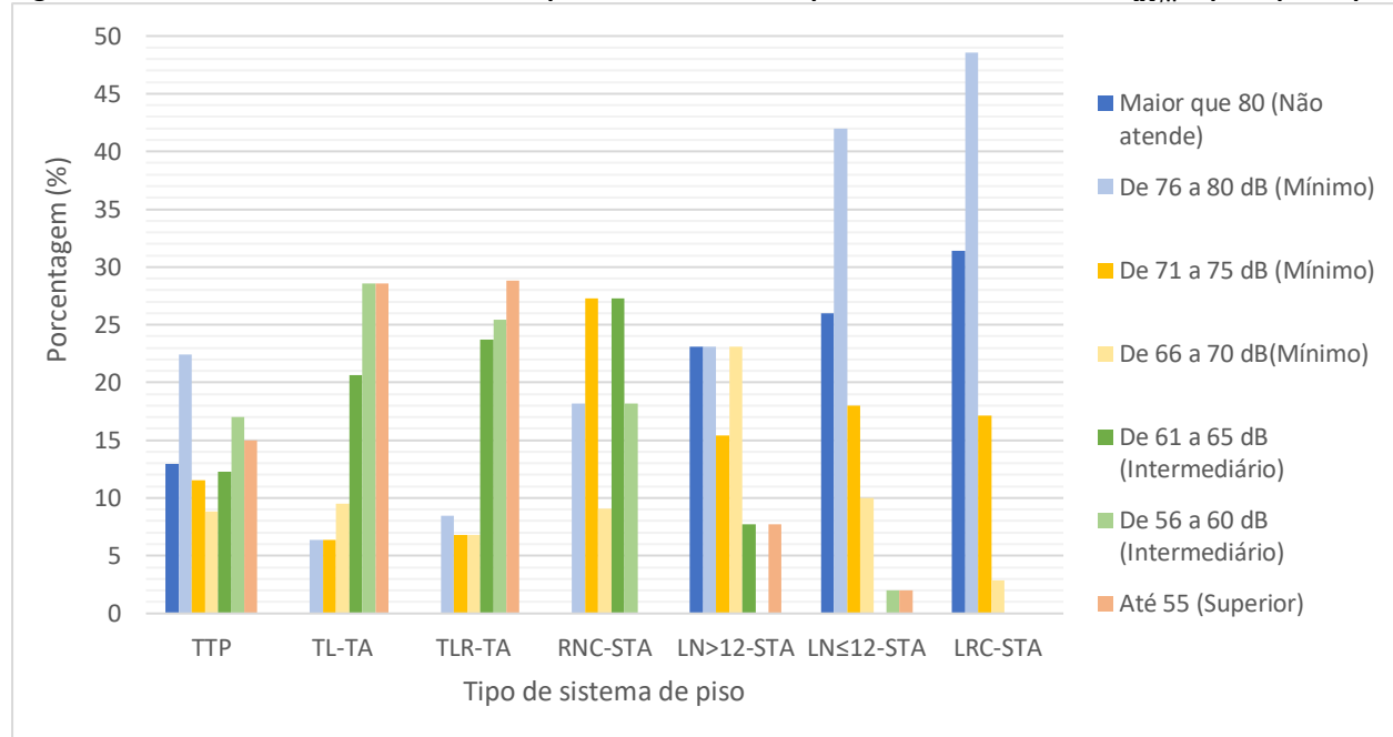
Figura 4: Atendimento ao critério de desempenho da NBR 15575 por faixas de valores de L'_{nT,w} e por tipo de piso
