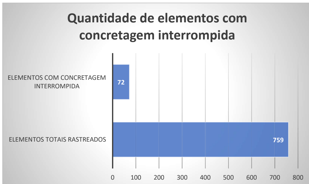
Gráfico 1 – Quantidade de elementos com concretagem interrompida
