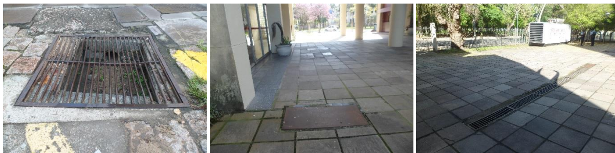
Figura 18: Grelha com aberturas e frestas largas (à esquerda) e caixas de inspeção e grelhas no fluxo principal de caminhamento (ao centro e à direita)
