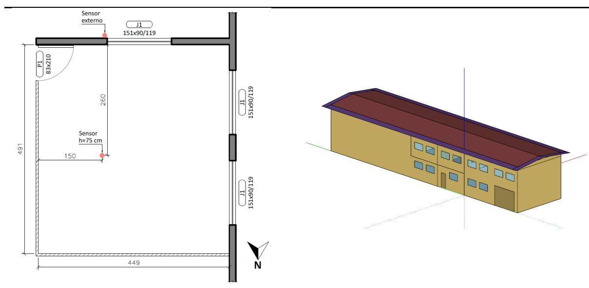
Figura 1: Planta esquemática da sala (à direita) e modelo tridimensional do edifício (à esquerda)
