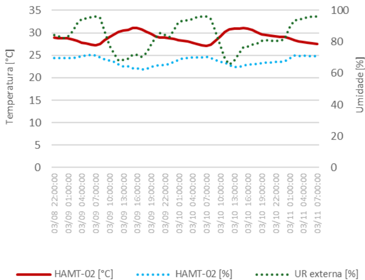
Figura 6: Temperatura e umidade internas, modelo HAMT com valores calculados de teor inicial de água
