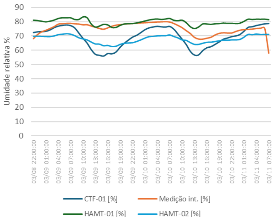
Figura 8: Umidade interna dos modelos numéricos e medição experimental
