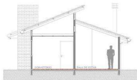
Figura 4. Corte BB da Casa Popular Eficiente – Sem escala
