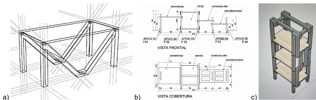
Figura 1: Concepção do projeto: a) croqui de mesa, b) desenho técnico de abrigo canino, c) modelo tridimensional de estante.
