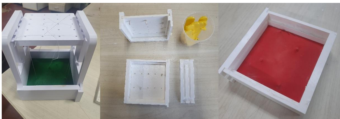
Figura 2: Primeiros dispositivos-moldes com incorporação de tecido (em verde) e borracha látex (em vermelho).
