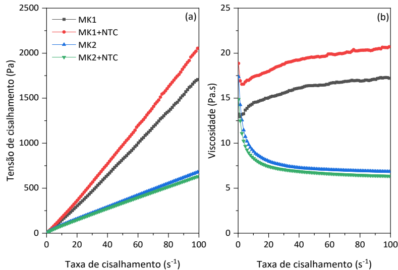
Figura 1 - Curvas de fluxo (a) e viscosidade vs. taxa de cisalhamento (b) das pastas geopoliméricas avaliadas
