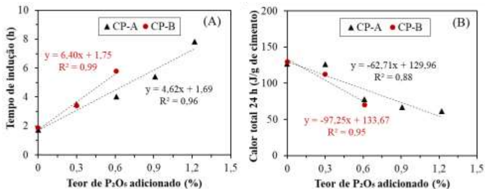
Figura 2: (A) Tempo de indução e (B) calor total liberado após 24 horas das pastas com diferentes teores de \text{P}_2\text{O}_5
