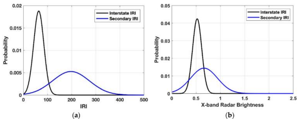
Figura 4 - Distribuição estatística dos valores do IRI para rodovias interestaduais (preto) e estradas secundárias (azul) em nossa área de estudo; (b) Distribuição estatística dos valores de brilho de radar pelos mesmos tipos de estradas.
