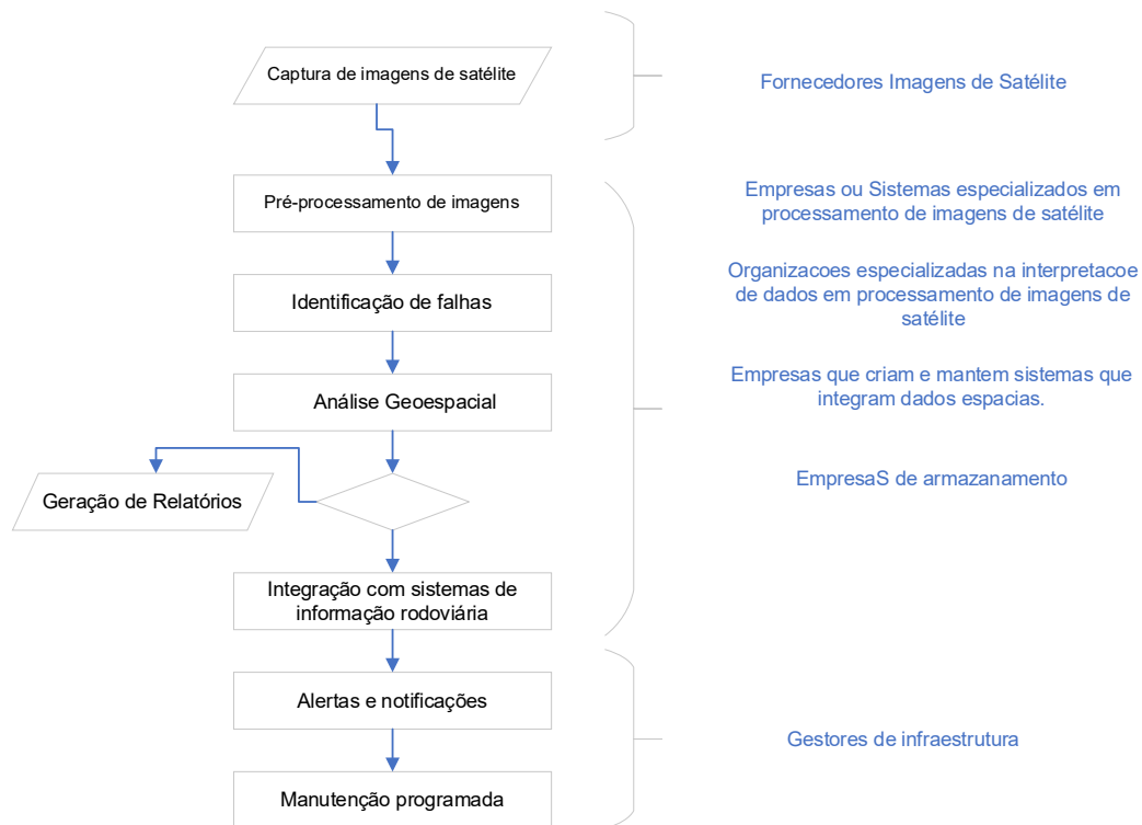
Figura 6 - Diagrama de fluxo dos processos para o monitoramento de pavimento asfáltico com a identificação dos agentes da cadeia produtiva
