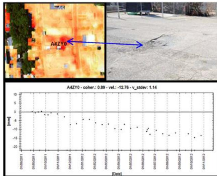
Figura 3 - Pavimento com deslocamento.
