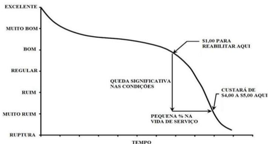
Figura 1 - Ciclo de vida de uma seção de pavimento.
