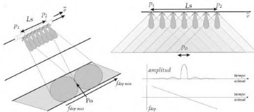
Figura 5 - Princípio de funcionamento do SAR
