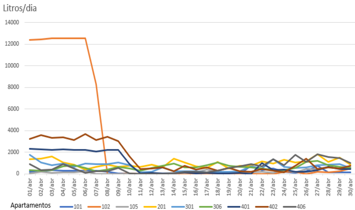
Figura 8 – Consumo diário de AF no mês de abril/2025.
