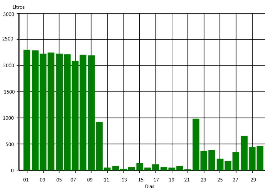
Figura 10 – Consumo diário de AF do apartamento 401, no mês de abril/2025.
