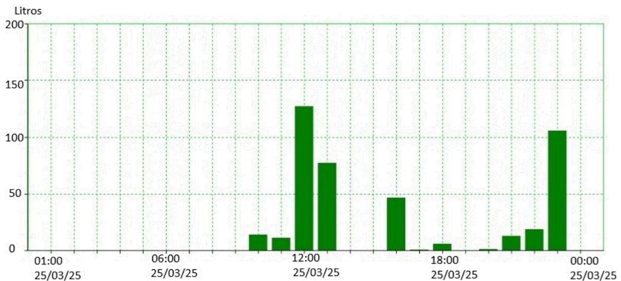
Figura 6 – Consumo horário total AF no Aptº 206, no dia 25/03/25.
