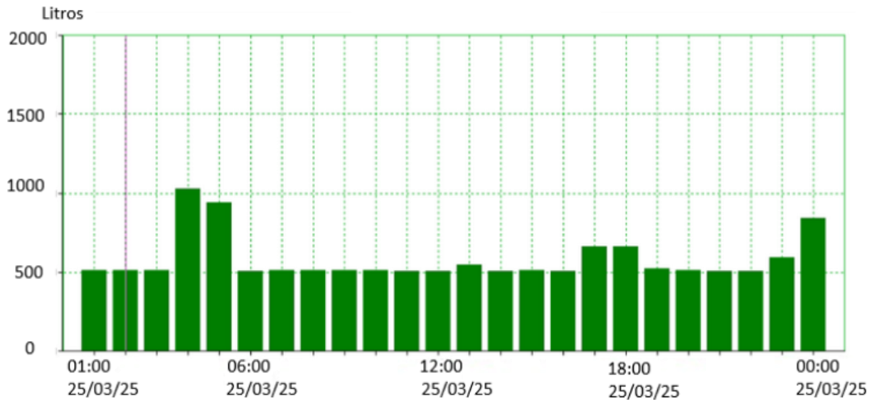
Figura 5 – Consumo horário total AF no Aptº 102, dia 25/03/25.
