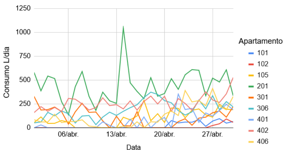
Figura 9 – Consumo diário de AQ no mês de abril/2025.
