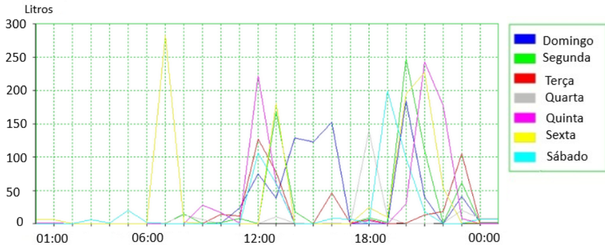
Figura 7 – Consumo horário de AF do apartamento 206 (semana de 23 a 29/03/25).
