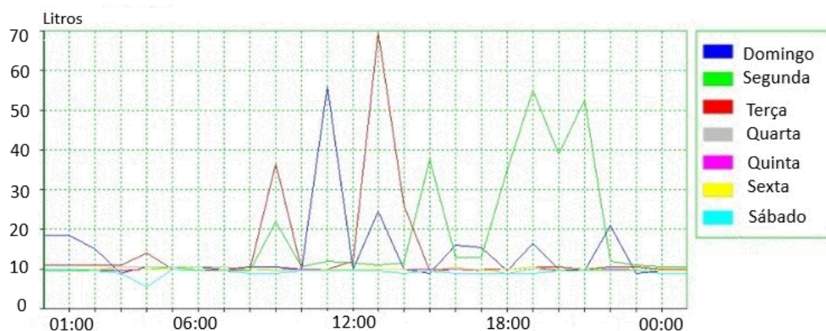
Figura 4 – Consumo horário de AF do apartamento 101 (semana de 23 a 29/03/25).
