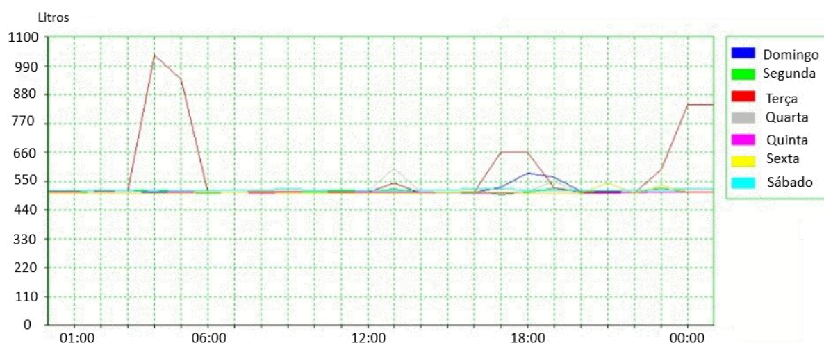
Figura 3 – Consumo horário de AF do apartamento 102 (semanal, de 23 a 29/03/25).
