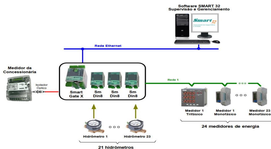
Figura 2 – Esquema Simplificado do Sistema de Telemetria na MUC
