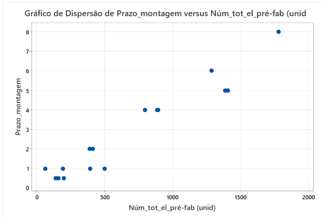
Gráfico 4: Dispersão de prazo de montagem (meses) versus número total de elementos pré-fabricados (unid)
