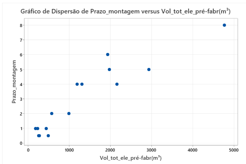
Gráfico 3: Dispersão de prazo de montagem (meses) versus volume total de elementos pré-fabricados (m 3 )
