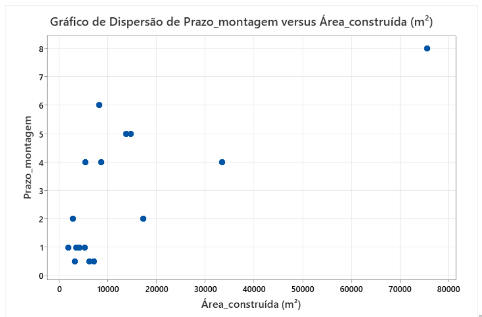
Gráfico 1: Dispersão de prazo de montagem (meses) versus área construída (m 2 )
